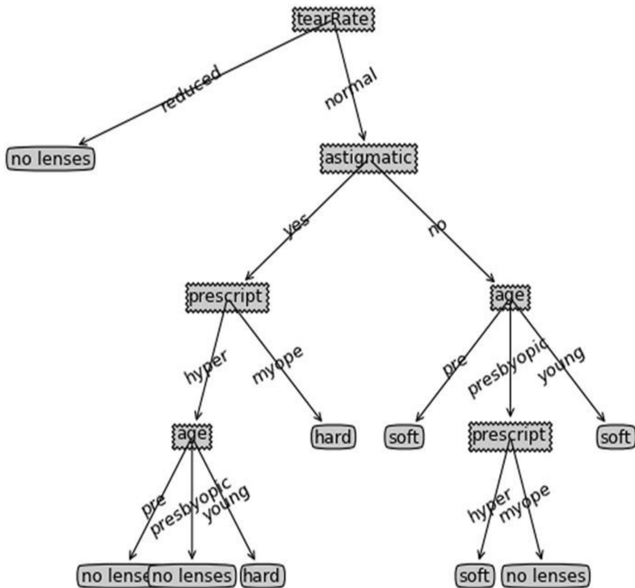
图3-8 由ID3算法产生的决策树
