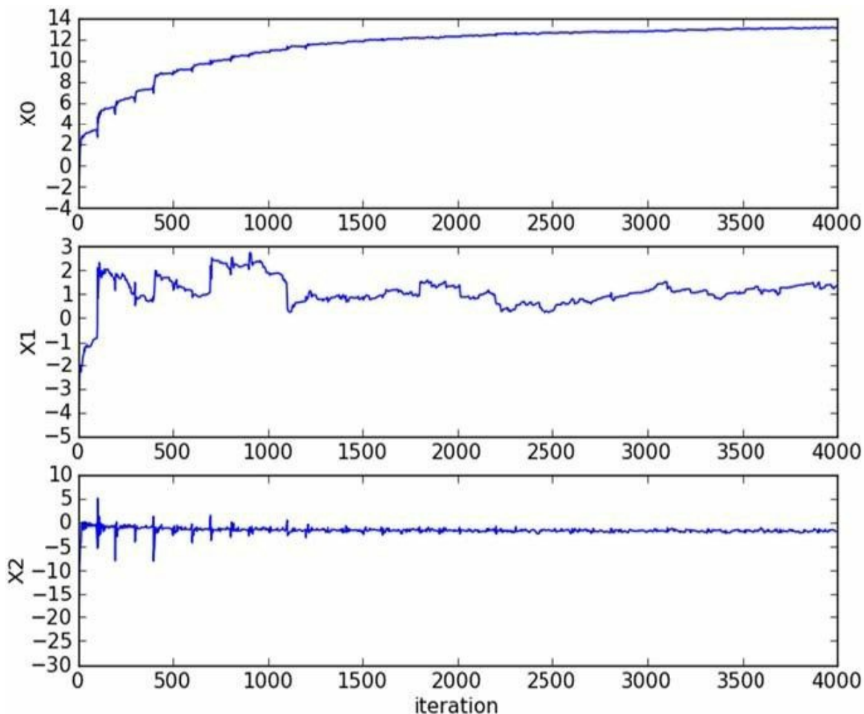
图5-7 使用样本随机选择和 \alpha 动态减少机制的随机梯度上升算法 stocGradAscent1() 所生成的系数收敛示意图。该方法比采用固定 \alpha 的方法收敛速度更快
