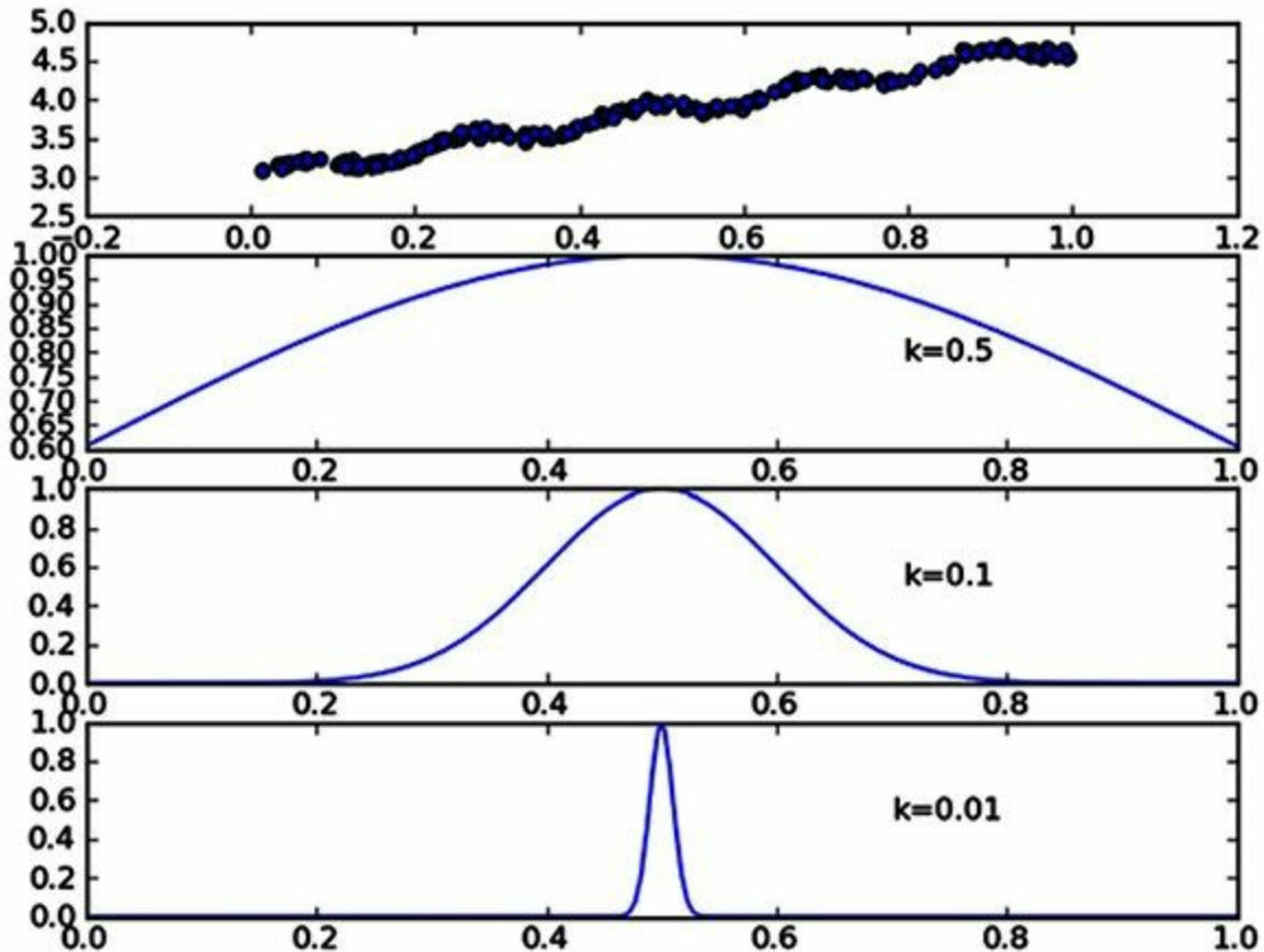
图8-4 每个点的权重图（假定我们正预测的点是 x = 0.5 ），最上面的图是原始数据集，第二个图显示了当 k = 0.5 时，大部分的数据都用于训练回归模型；而最下面的图显示当 k = 0.01 时，仅有很少的局部点被用于训练回归模型
