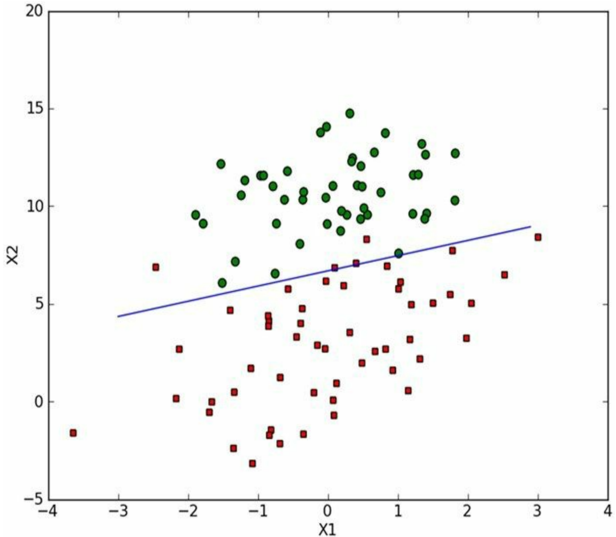
图5-4 梯度上升算法在500次迭代后得到的Logistic回归最佳拟合直线
