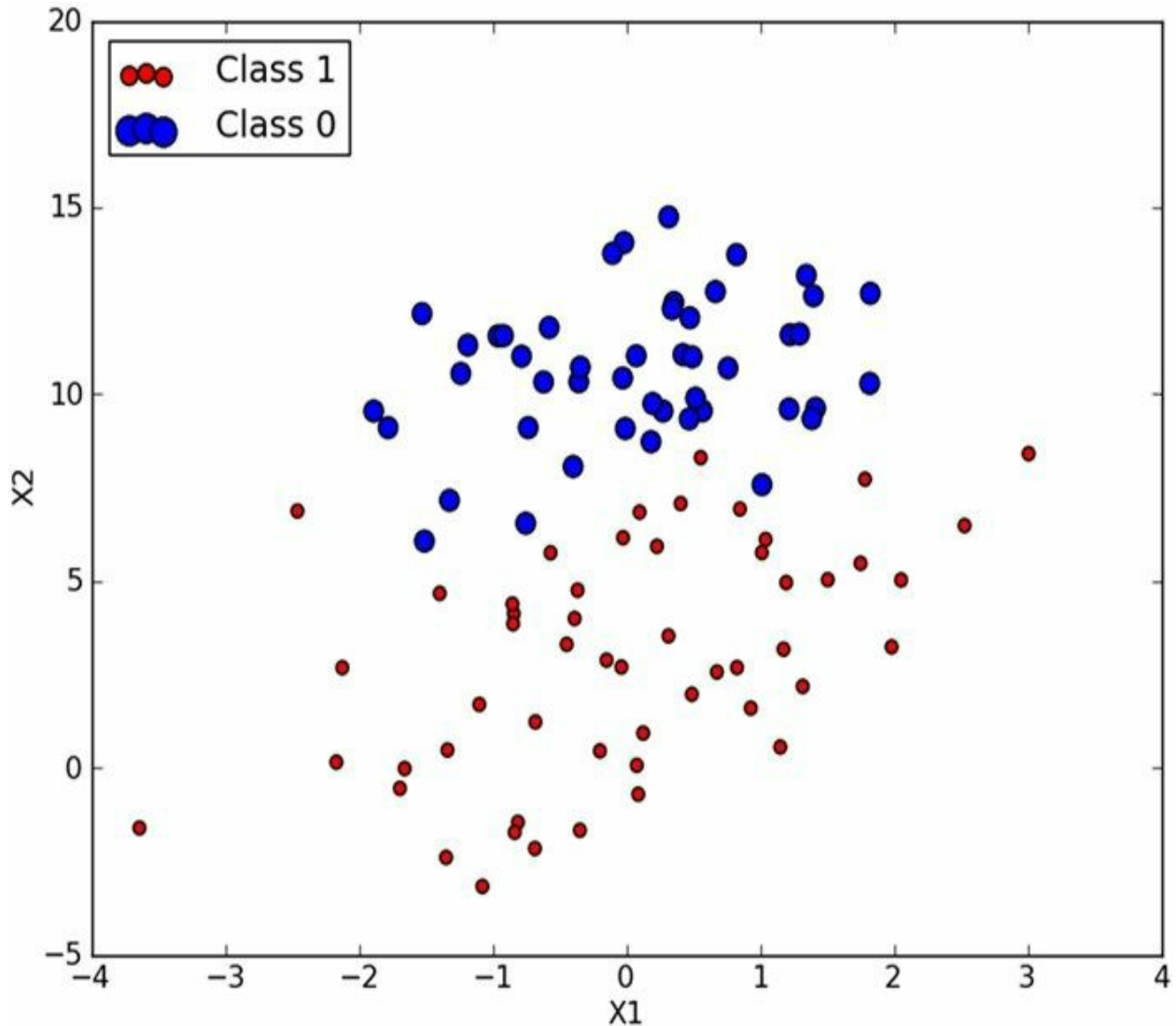
图5-3 一个简单数据集，下面将采用梯度上升法找到 Logistic 回归分类器在此数据集上的最佳回归系数
