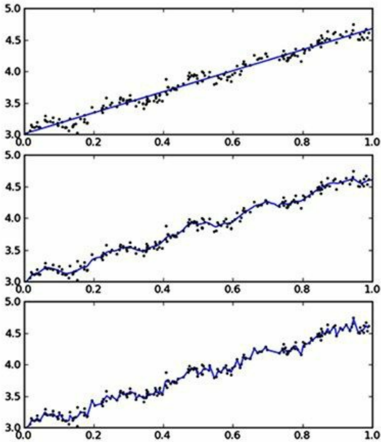
图8-5 使用3种不同的平滑值绘出的局部加权线性回归结果。上图中的平滑参数 k = 1.0 ，中图 k = 0.01 ，下图 k = 0.003 。可以看到， k = 1.0 时的模型效果与最小二乘法差不多， k = 0.01 时该模型可以挖出数据的潜在规律，而 k = 0.003 时则考虑了太多的噪音，进而导致了过拟合现象
