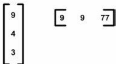
图B-2 左边给出了一个列向量，右边给出了一个行向量
