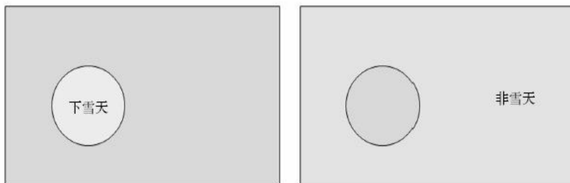
图C-1 上图的圆圈内表示“下雪天”事件（将其他事件排除在圆圈之外），下图的圆圈外则表示除“雪天”外的其他所有事件。这样，雪天和非雪天就包括了所有事件。
