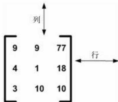
图B-1 一个简单的3x3矩阵，图中给出了行、列的方向
