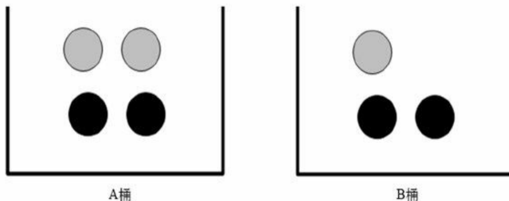
图4-3 落到两个桶中的7块石头
