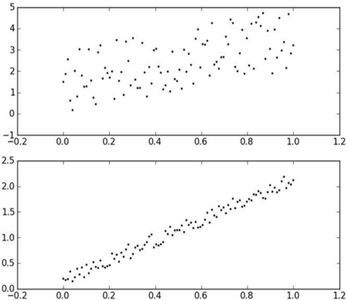
图8-3 具有相同回归系数（ 0 和 2.0 ）的两组数据。上图的相关系数是 0.58 ，而下图的相关系数是 0.99
