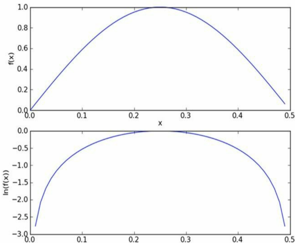
图4-4 函数 f(x) 与 \ln(f(x)) 会一块增大。这表明想求函数的最大值时，可以使用该函数的自然对数来替换原函数进行求解
