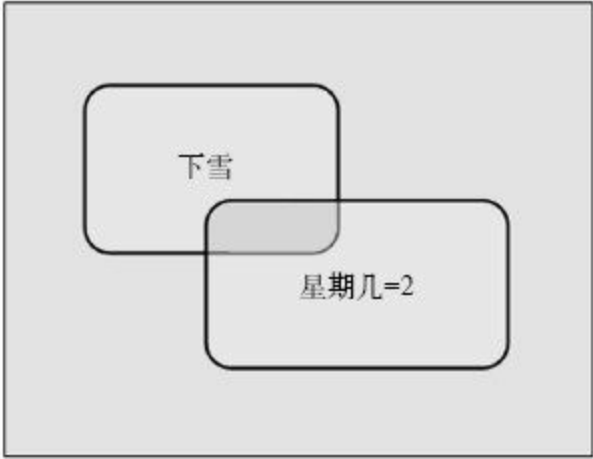
图C-2 表示两个相交事件的文氏图
