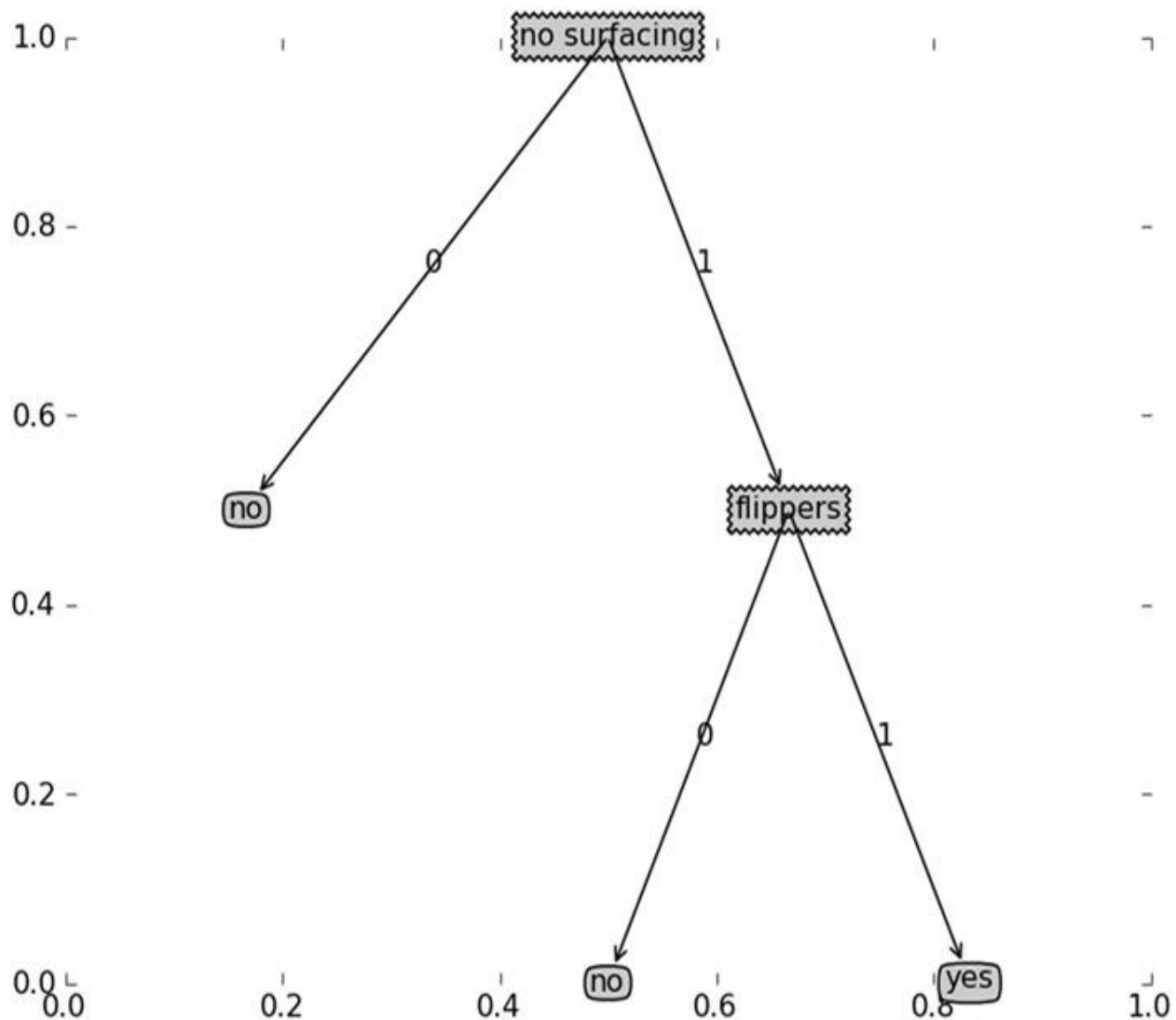
图3-6 简单数据集绘制的树形图
