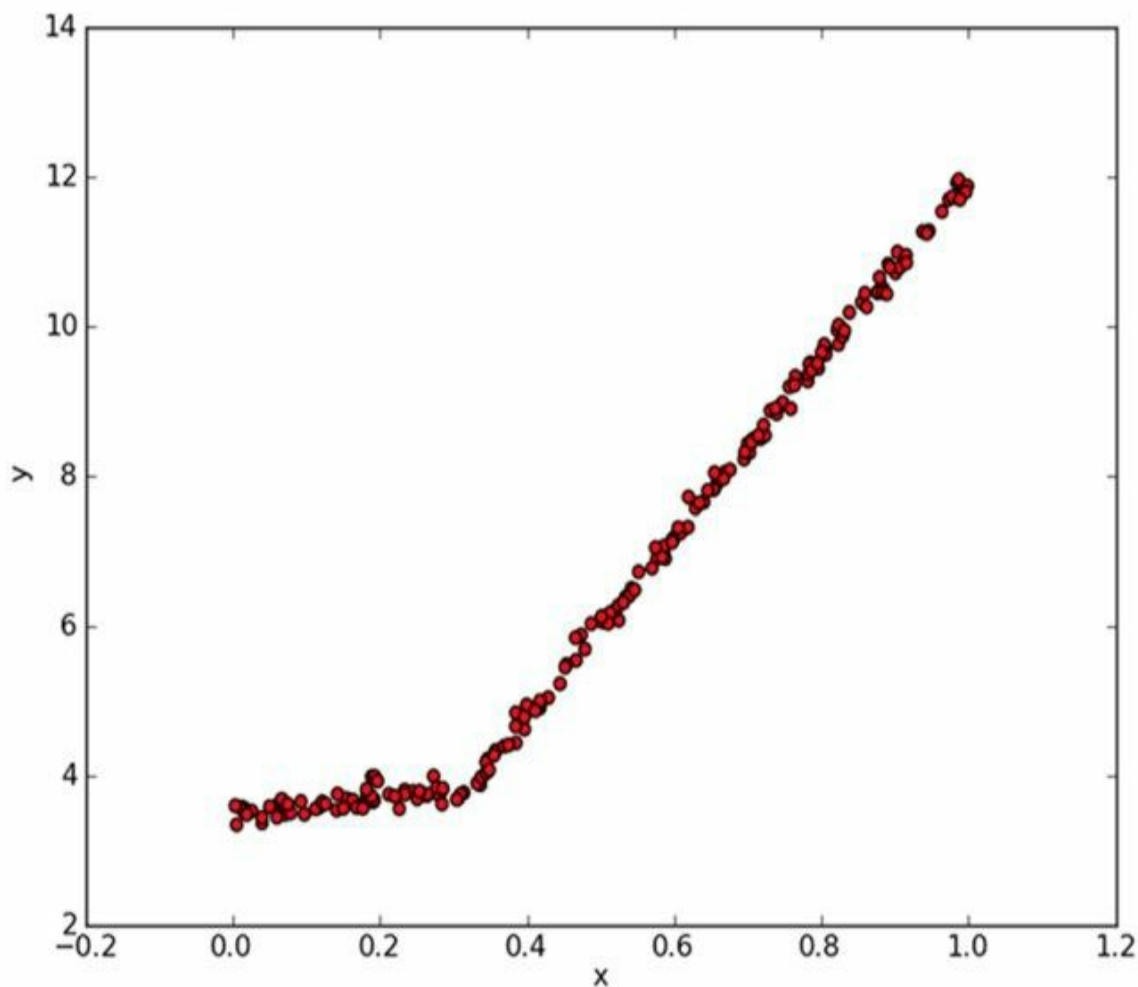
图9-4 用来测试模型树构建函数的分段线性数据
