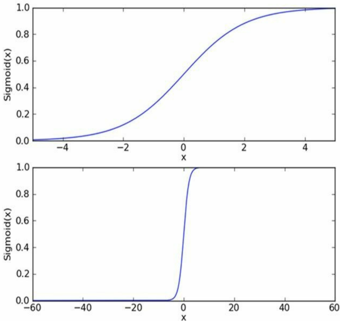
图5-1 两种坐标尺度下的 Sigmoid 函数图。上图的横坐标为-5到5，这时的曲线变化较为平滑；下图横坐标的尺度足够大，可以看到，在 x = 0 点处 Sigmoid 函数看起来很像阶跃函数
