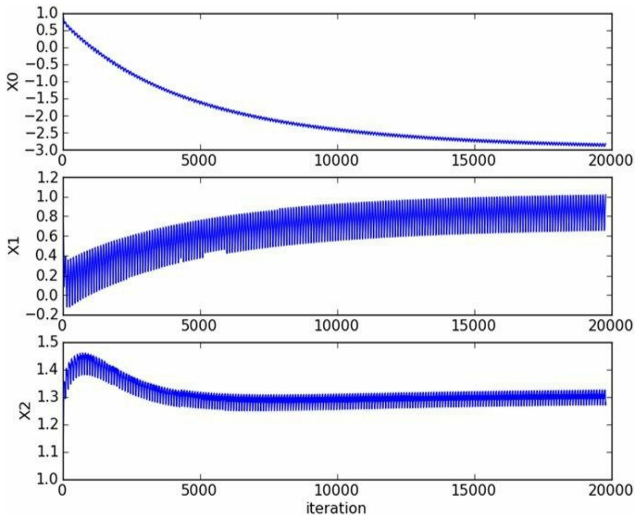
图5-6 运行随机梯度上升算法，在数据集的一次遍历中回归系数与迭代次数的关系图。回归系数经过大量迭代才能达到稳定值，并且仍然有局部的波动现象
