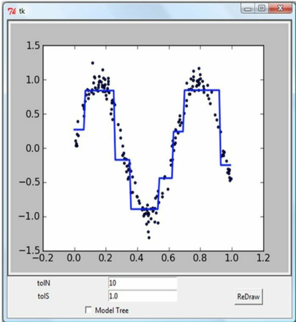
图9-7 默认的treeExplore图形用户界面，该界面同时显示了输入数据和一个回归树模型，其中的参数tolN = 10，tolS = 1.0
