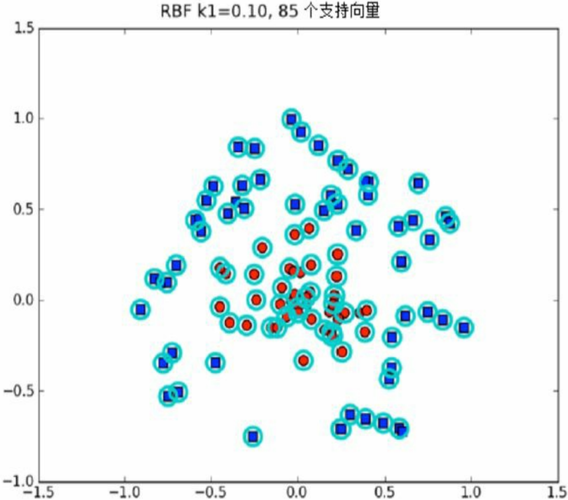
图6-7 在用户自定义参数 k_1 = 0.1 时的径向基函数。该参数此时减少了每个支持向量的影响程度，因此需要更多的支持向量
