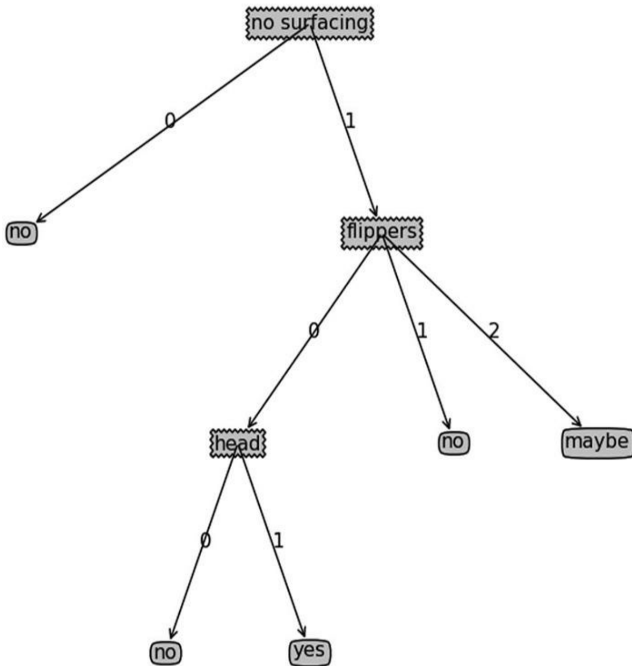
图3-3 决策树的范例
