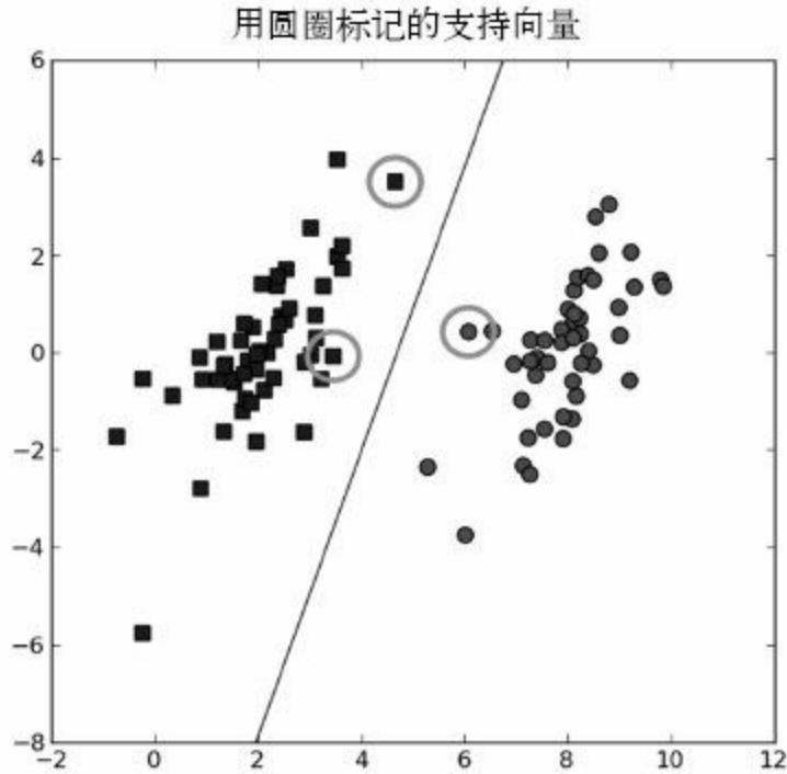
图6-4 在示例数据集上运行简化版SMO算法后得到的结果，包括画圈的支持向量与分隔超平面
