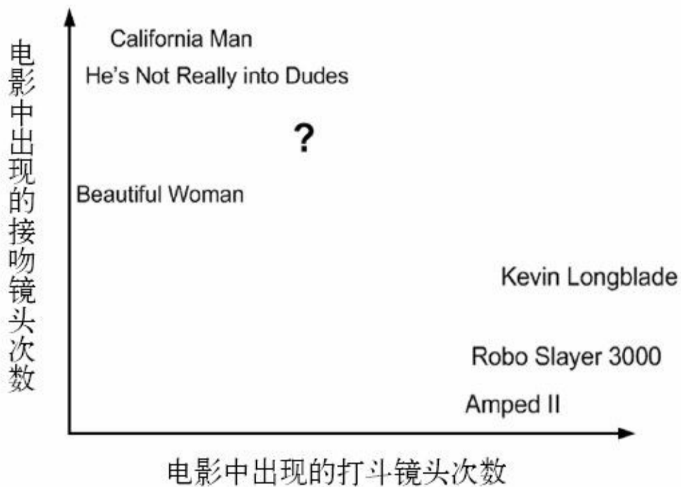
图2-1 使用打斗和接吻镜头数分类电影
