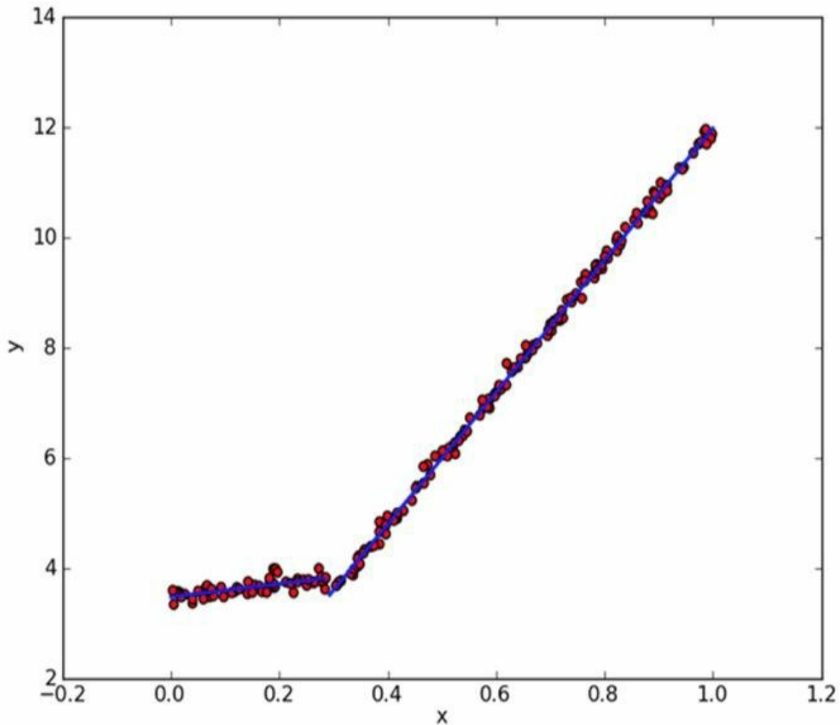
图9-5 在图9-4数据集上应用模型树算法得到的结果
