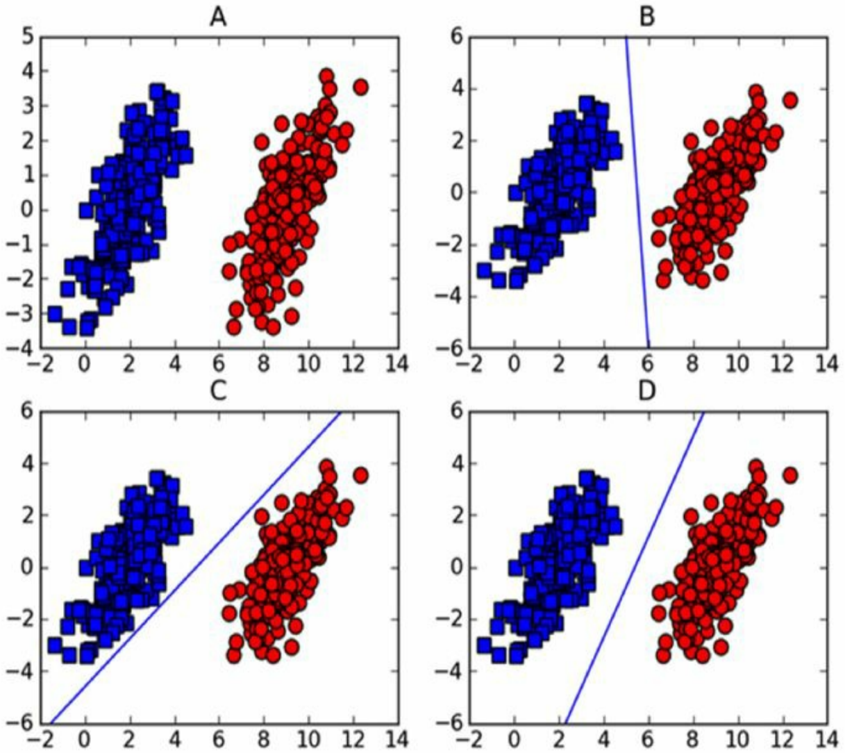
图6-2 A框中给出了一个线性可分的数据集，B、C、D框中各自给出了一条可以将两类数据分开的直线
