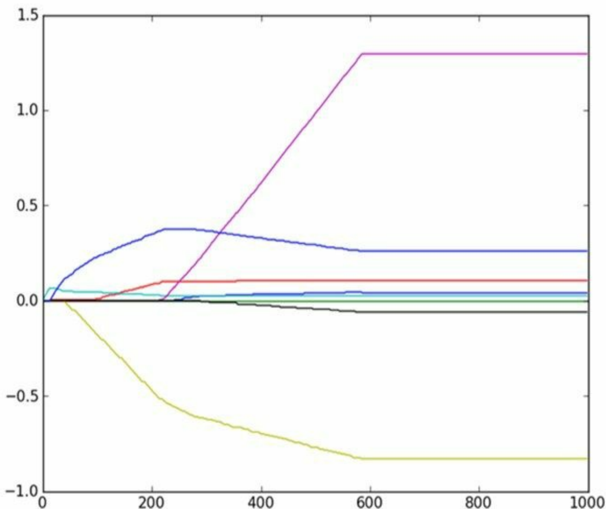
图8-7 鲍鱼数据集上执行逐步线性回归法得到的系数与迭代次数间的关系。逐步线性回归得到了与lasso相似的结果，但计算起来更加简便
