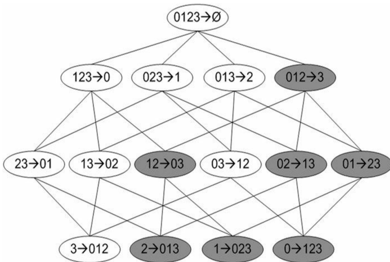
图11-4 对于频繁项集{0,1,2,3}的关联规则网格示意图。阴影区域给出的是低可信度的规则。如果发现0,1,2 → 3是一条低可信度规则，那么所有其他以3作为后件的规则可信度也会较低
