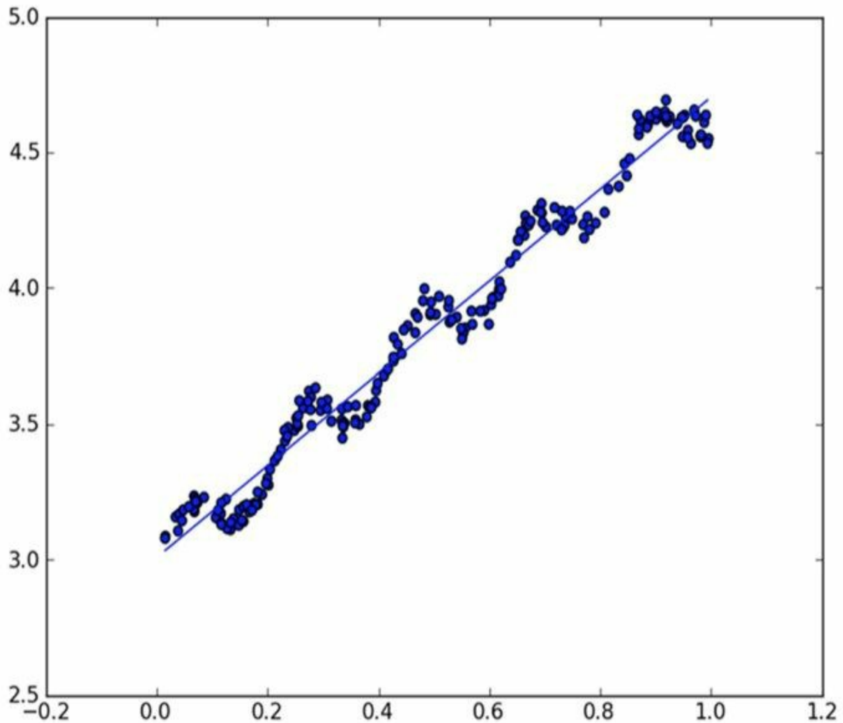
图8-2 ex0.txt 的数据集与它的最佳拟合直线
