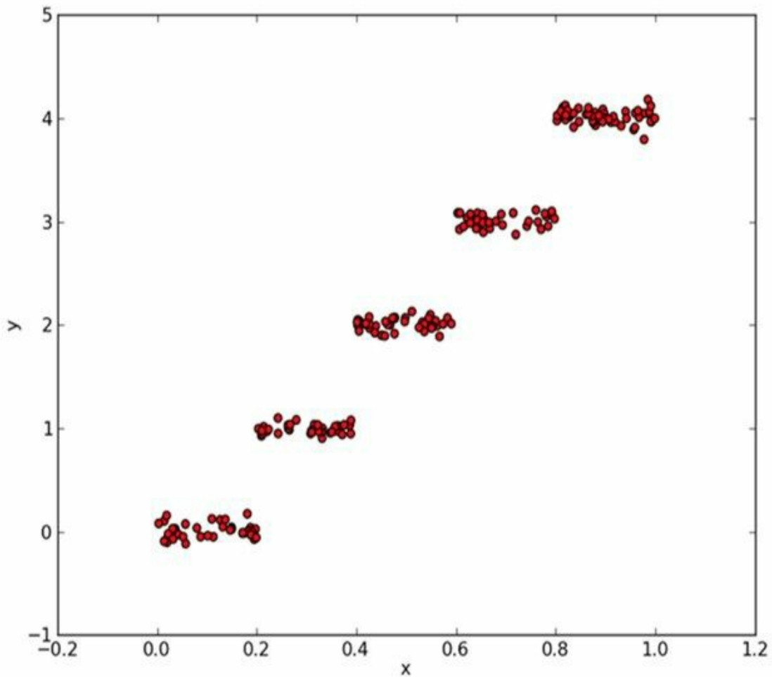
图9-2 用于测试回归树的分段常数数据集
