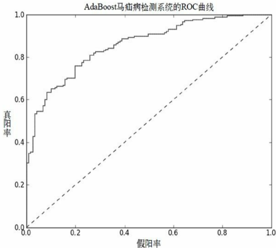
图7-3 利用10个单层决策树的AdaBoost马疝病检测系统的ROC曲线
