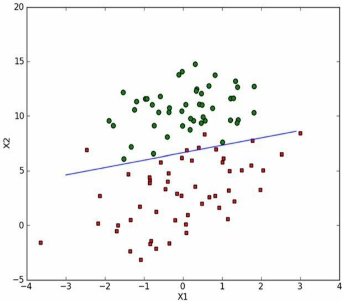
图5-8 使用改进的随机梯度上升算法得到的系数
