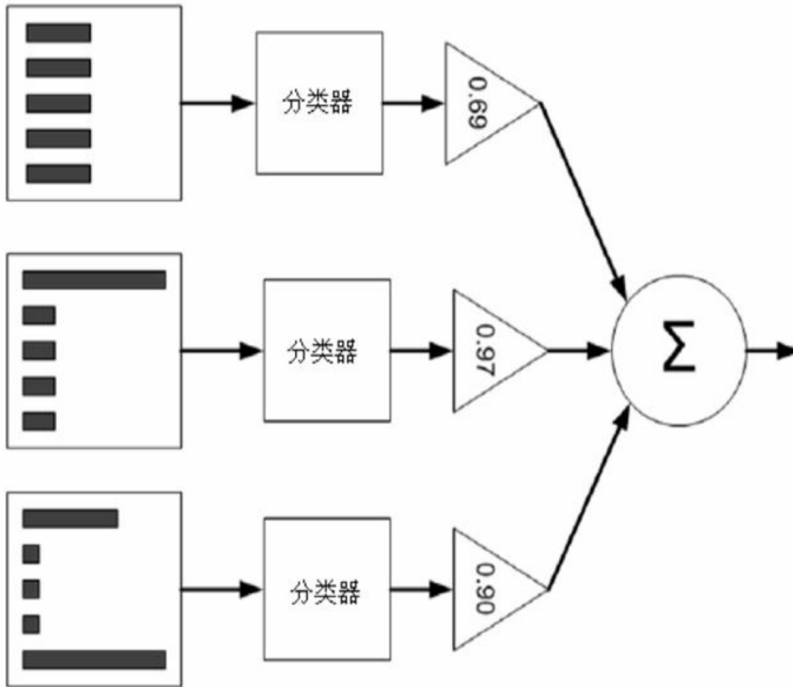
图7-1 AdaBoost算法的示意图。左边是数据集，其中直方图的不同宽度表示每个样例上的不同权重。在经过一个分类器之后，加权的预测结果会通过三角形中的 \alpha 值进行加权。每个三角形中输出的加权结果在圆形中求和，从而得到最终的输出结果
