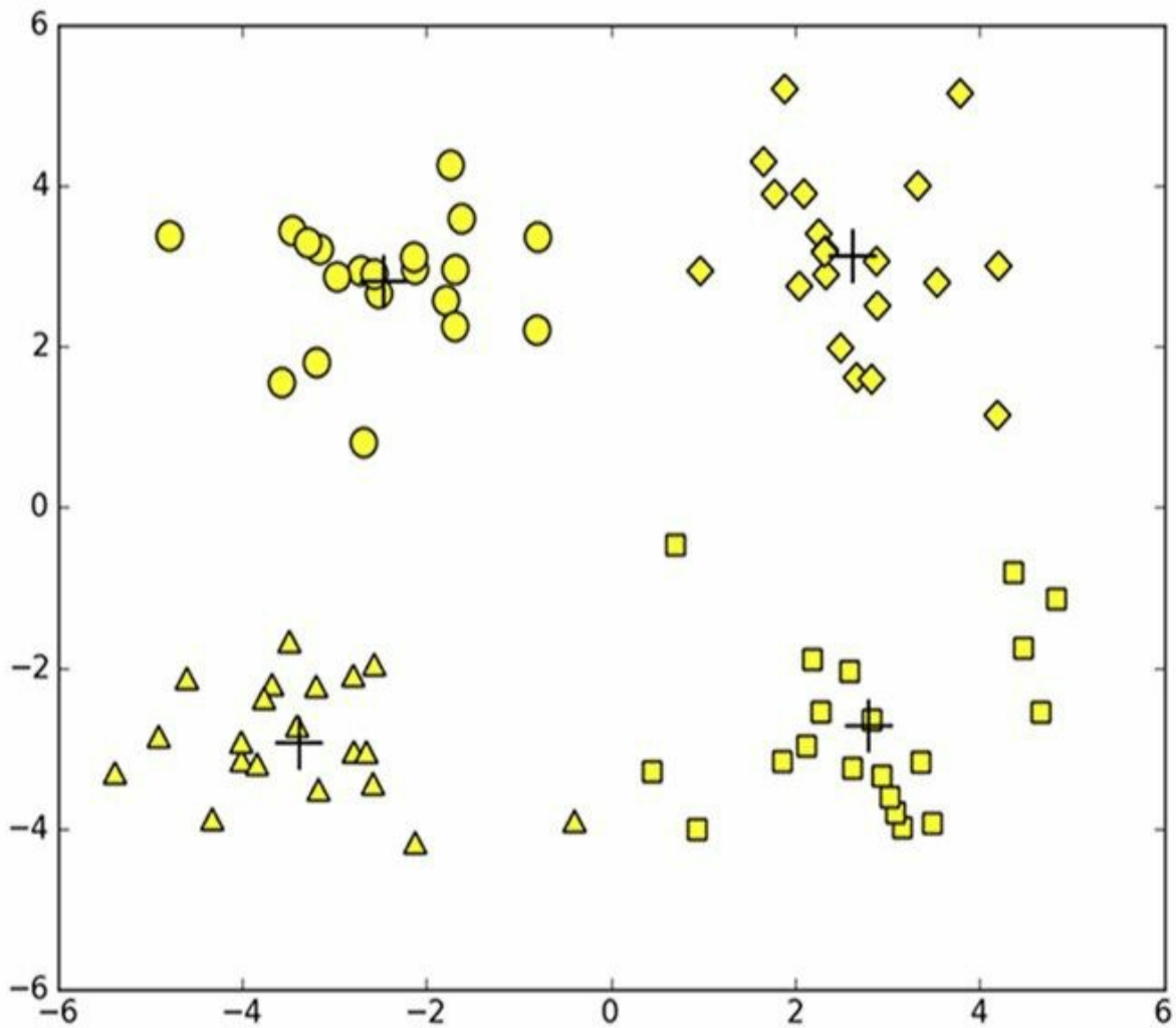
图10-1 k均值聚类的结果示意图。图中数据集在三次迭代之后收敛。形状相似的数据点被分到同样的簇中，簇中心使用十字来表示
