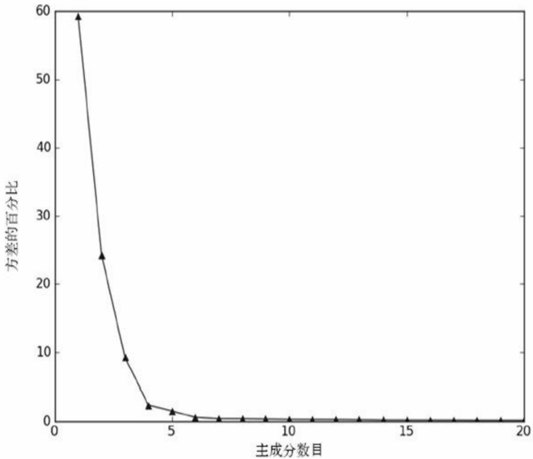
图13-4 前20个主成分占总方差的百分比。可以看出，大部分方差都包含在前面的几个主成分中，舍弃后面的主成分并不会损失太多的信息。如果保留前6个主成分，则数据集可以从590个特征约简成6个特征，大概实现了100:1的压缩
