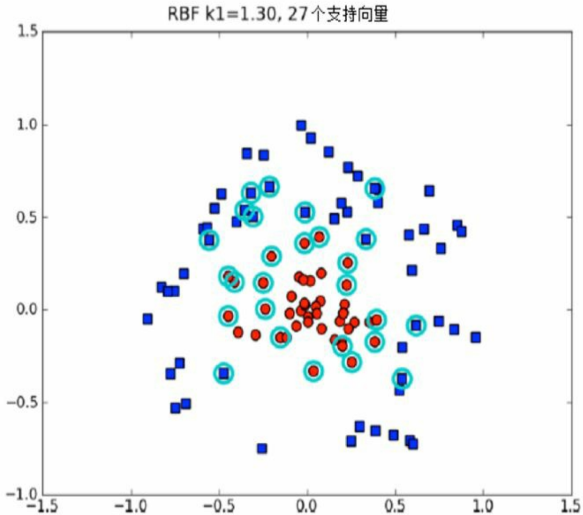
图6-8 在用户自定义参数 k1=1.3 时的径向基函数。这里的支持向量个数少于图6-7的，而这些支持向量在决策边界周围聚集
