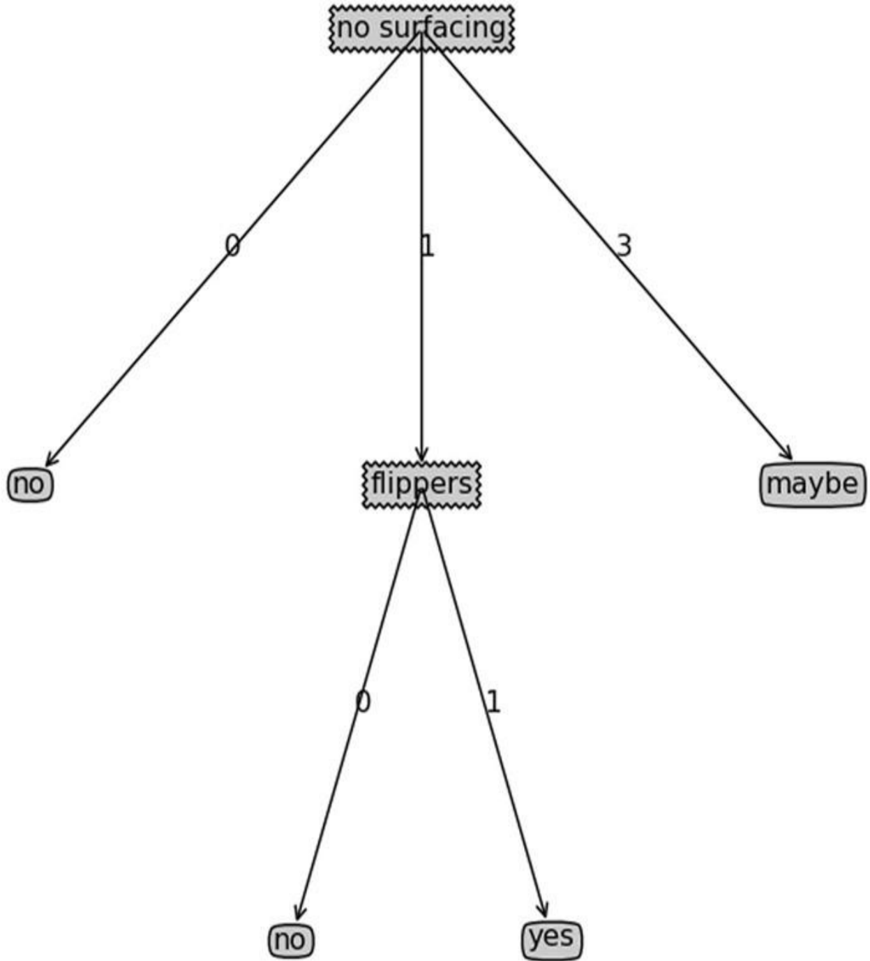
图3-7 超过两个分支的树形图
