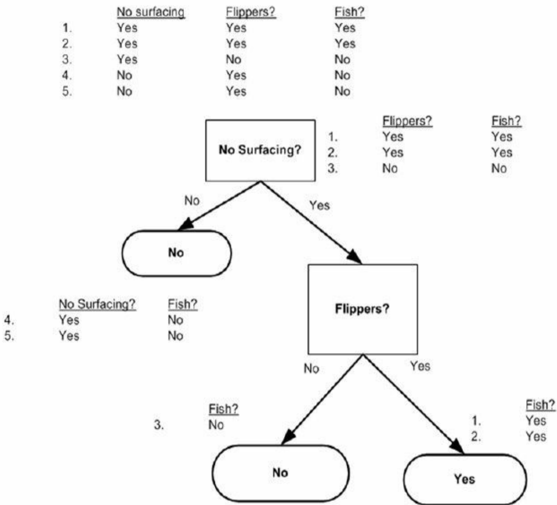
图3-2 划分数据集时的数据路径
