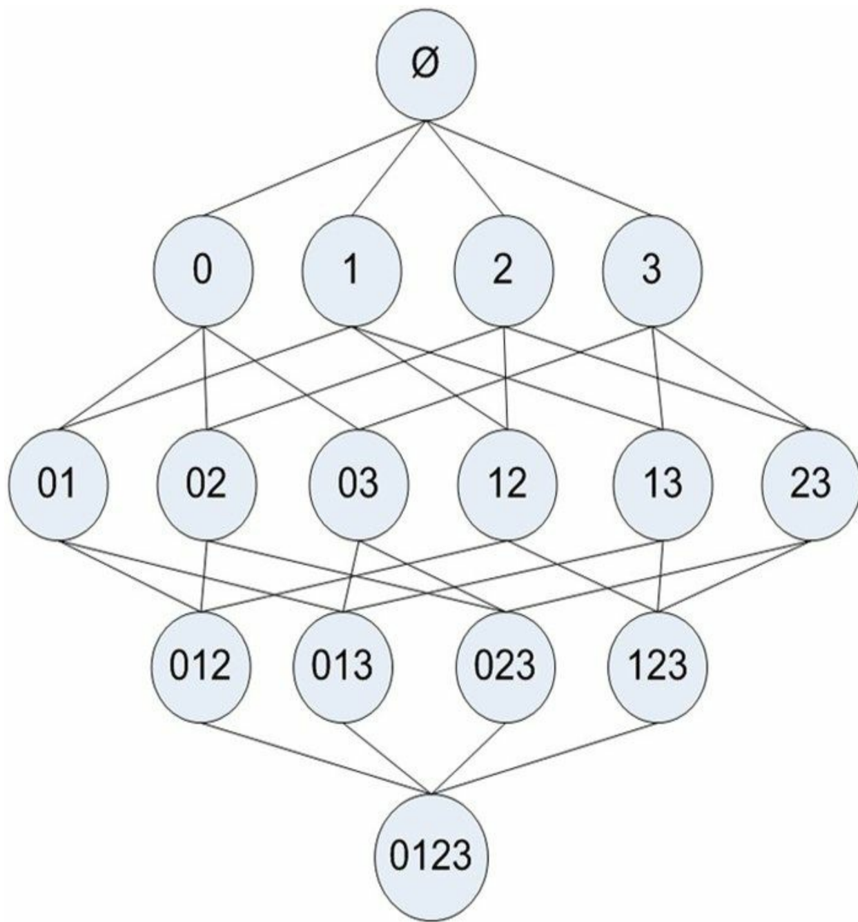
图11-2 集合{0,1,2,3}中所有可能的项集组合
