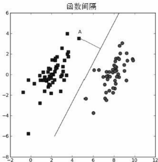
图6-3 A到分隔平面的距离就是该点到分隔面的法线长度
